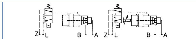
Ventil spannungslos Ruhestellung (geschlossen)
