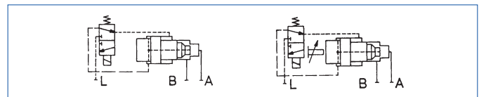
Ventil spannungslos Ruhestellung ( geschlossen )
