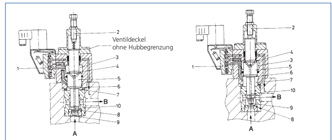
Ventil spannungslos Ruhestellung ( geschlossen )
