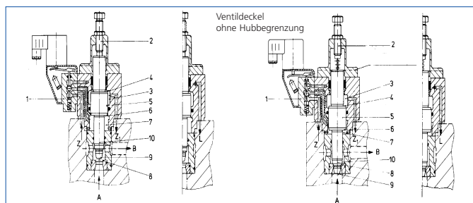
Ventil spannungslos (Ruhestellung (geöffnet)
