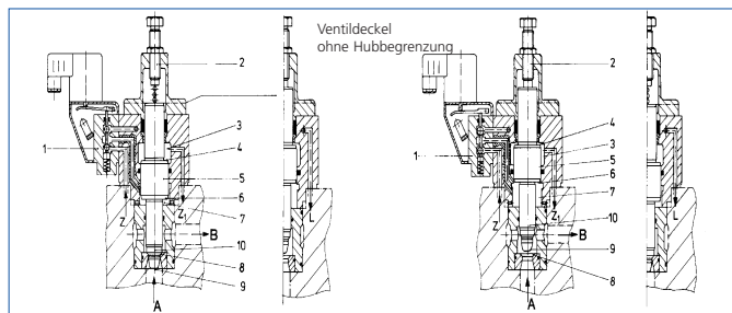
Ventil spannungslos Ruhestellung (geschlossen)
